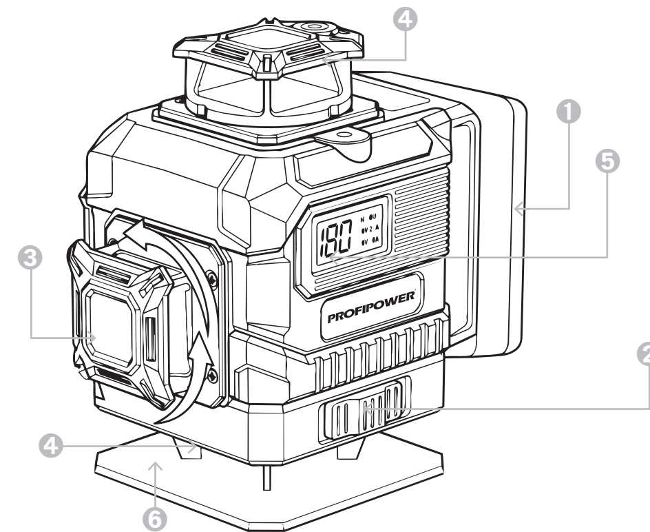
Рисунок 1.5. Устройство инструмента
